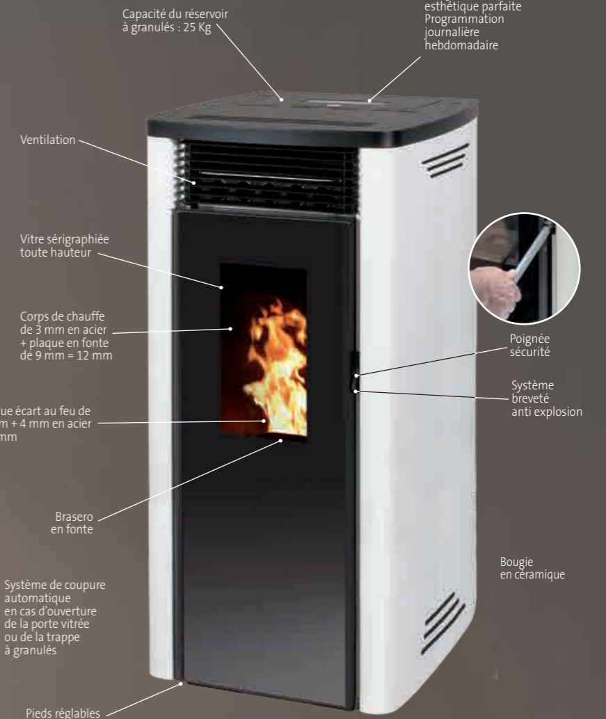
Pieds réglables
